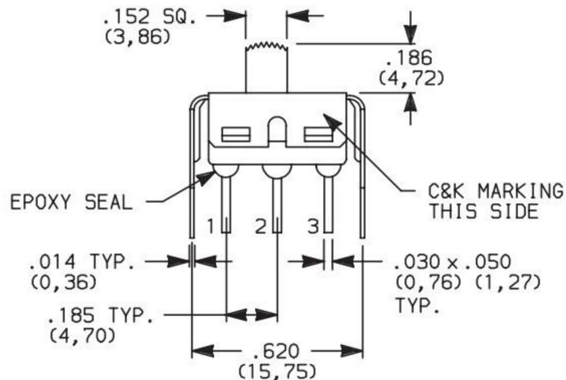
Actuator Shown In Pos. 1
